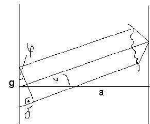
Abbildung 1: Beugung von Licht am Doppelspalt
