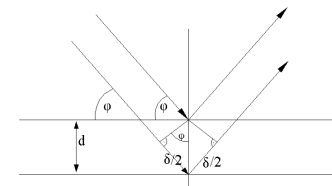
Abbildung 2: Reflexion von Röntgenstrahlen am Kristallgitter
